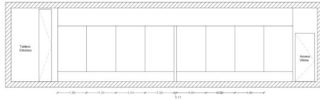
CORTE A-A' ELEVACIÓN FRONTAL VITRINA
